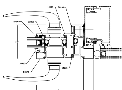
4B 112-4B OPTIONAL DS LOCK JAMB SSG
