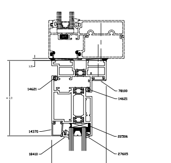
1 112-1 STANDARD DS HEAD FLAT
