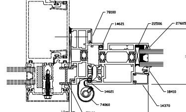
3A 112-3A OPTIONAL DS HINGE JAMB CAPTURED
