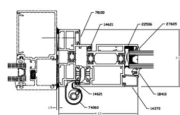
3 112-3 STANDARD DS HINGE JAMB FLAT
