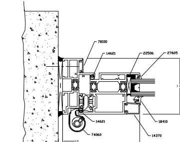
3C 112-3C OPTIONAL DS HINGE JAMB
