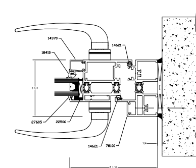
8C 112-8C OPTIONAL IS LOCK JAMB
