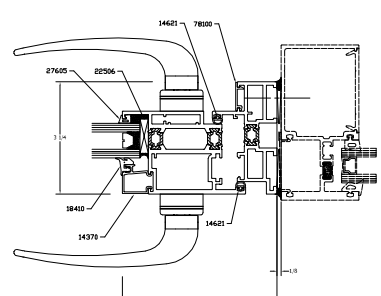
4 112-4 STANDARD DS LOCK JAMB FLAT
