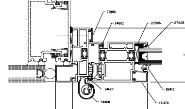
3B 112-3B OPTIONAL DS HINGE JAMB SSG
