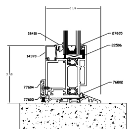
2A 112-2A OPTIONAL DS accessible SILL 12psf WATER ONLY
