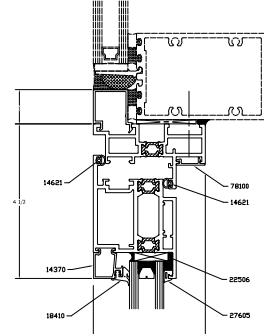
1B 112-1B OPTIONAL DS HEAD SSG
