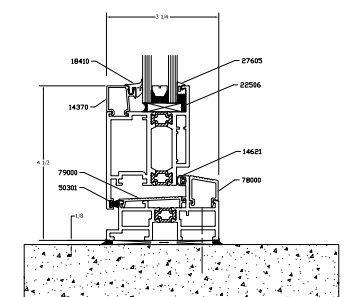
2 112-2 STANDARD DS SILL
