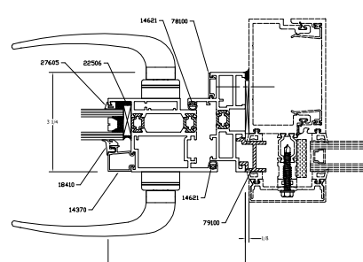
4A 112-4A OPTIONAL DS LOCK JAMB CAPTURED
