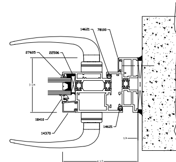
4C 112-4C OPTIONAL DS LOCK JAMB
