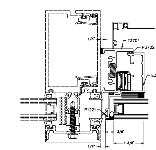
19A JAMB GLAZED-IN FRAME OPTIONAL
