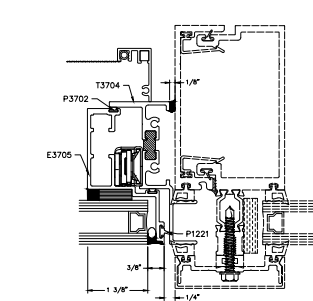
20A JAMB GLAZED-IN FRAME OPTIONAL
