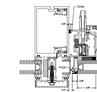
23A JAMB GLAZED-IN FRAME OPTIONAL
