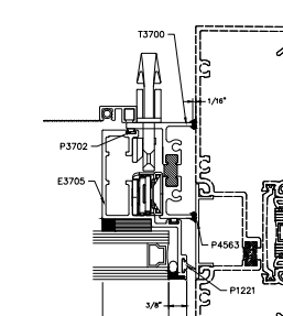
24B JAMB SF ADAPTER OPTIONAL
