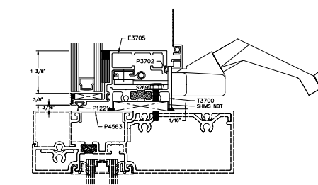
22B SILL SF ADAPTER OPTIONAL
