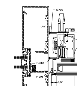
23B JAMB SF ADAPTER OPTIONAL
