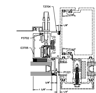
24A JAMB GLAZED-IN FRAME OPTIONAL
