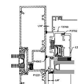
19B JAMB SF ADAPTER OPTIONAL
