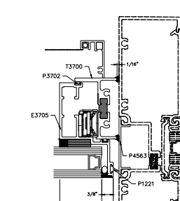
20B JAMB SF ADAPTER OPTIONAL
