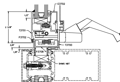
14A SILL CW ADAPTER OPTIONAL
