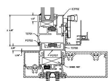
10B SILL SF ADAPTER OPTIONAL
