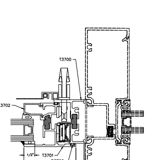
16B JAMB SF ADAPTER OPTIONAL
