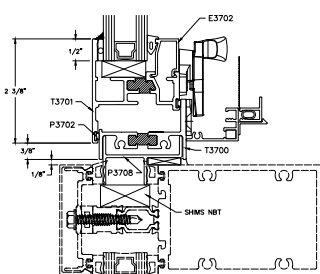
10A SILL CW ADAPTER OPTIONAL
