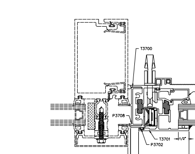
15A JAMB CW ADAPTER OPTIONAL
