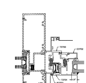
11B JAMB SF ADAPTER OPTIONAL
