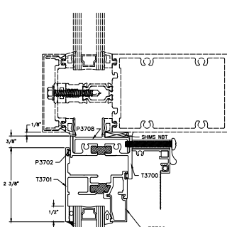
9A HEAD CW ADAPTER OPTIONAL
