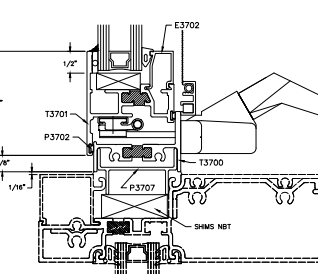
14B SILL SF ADAPTER OPTIONAL
