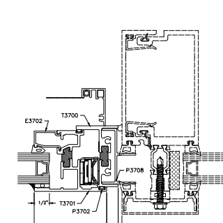
12A JAMB CW ADAPTER OPTIONAL
