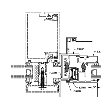
11A JAMB CW ADAPTER OPTIONAL
