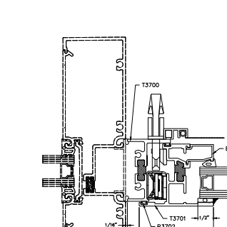
15B JAMB SF ADAPTER OPTIONAL
