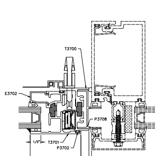
16A JAMB CW ADAPTER OPTIONAL
