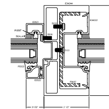
6A OPTIONAL HD DEEP POCKET TRANSOM JAMB
