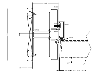
8A STANDARD HD DOOR JAMB
