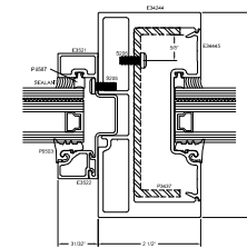
6 STANDARD HD TRANSOM JAMB
