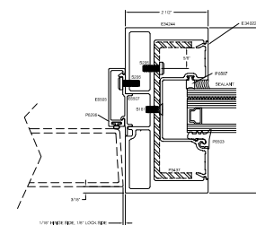
9A OPTIONAL HD INT. DOOR JAMB DEEP POCKET
