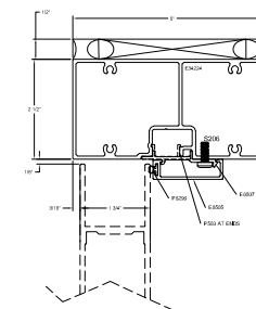
7B OPTIONAL NO TRANSOM DOOR HEAD
