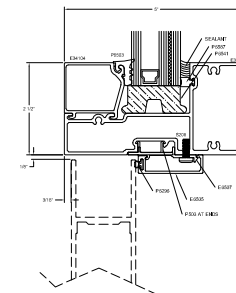
7 STANDARD DOOR HEADER
