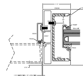
9 STANDARD HD INT. DOOR JAMB
