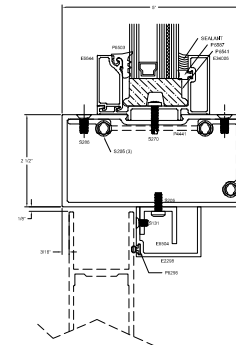
7A OPTIONAL DOOR HEADER
