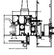
4B JAMB SF INSTALLATION OPTIONAL
