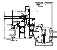
8A JAMB CURTAIN WALL INSTALLATION OPTIONAL
