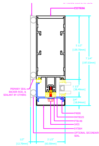
5 STANDARD TUBULAR JAMB
