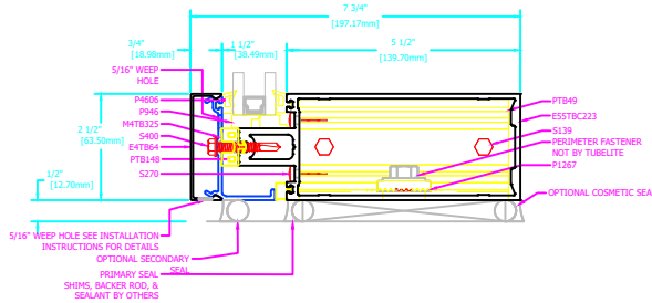
3 STANDARD TUBULAR SILL
