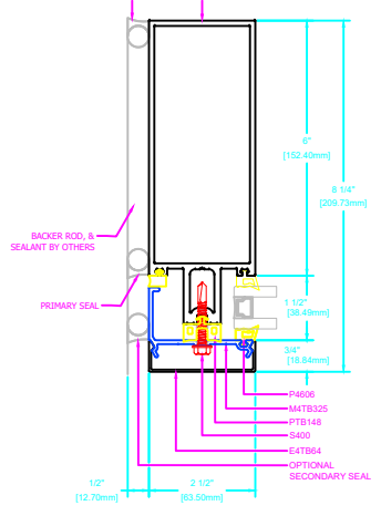
5 STANDARD TUBULAR JAMB
